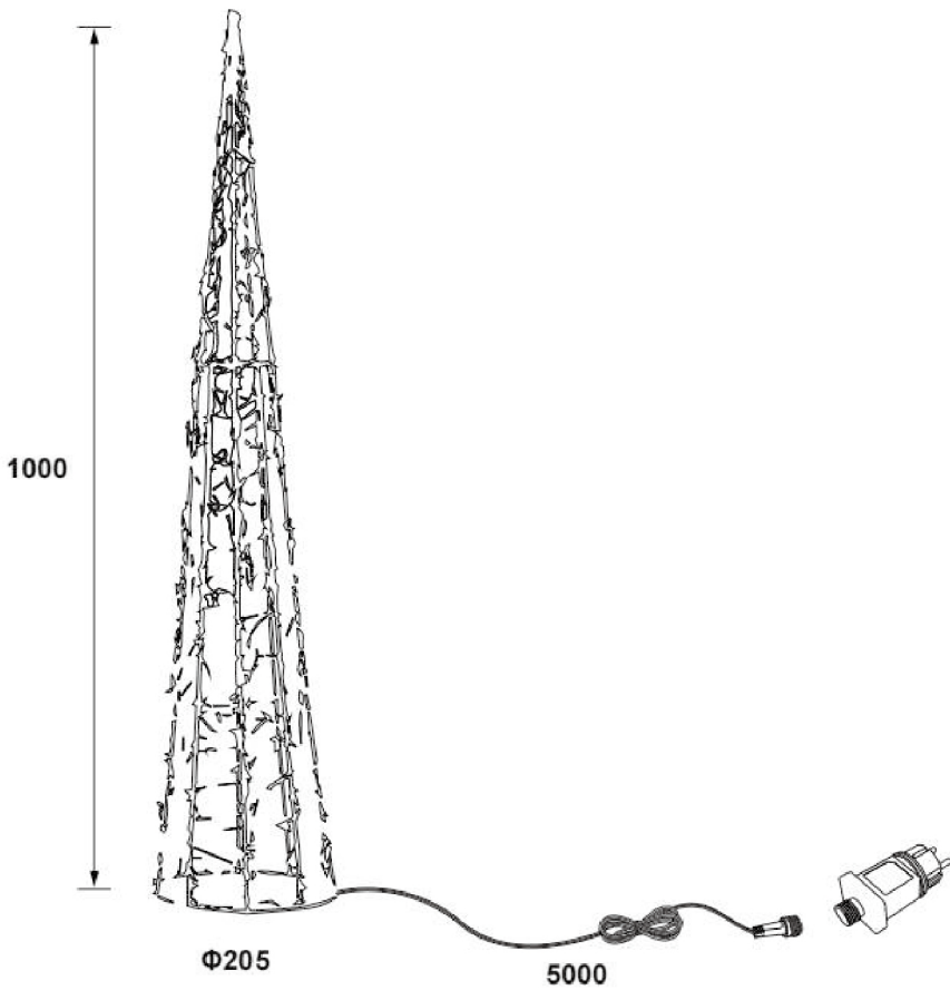
Unit of measure/ Maßeinheit/ Unité de mesure: mm
